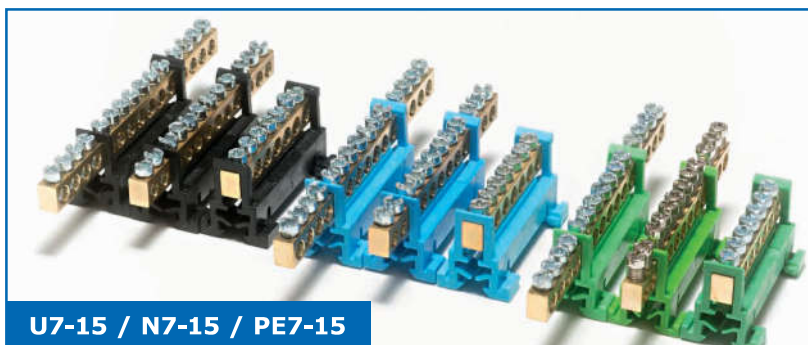
PE/N-kiskojeen Cu-syöttöliitin.
